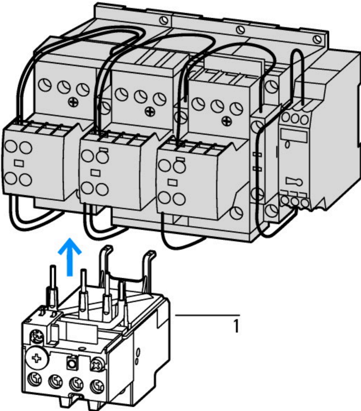
1: Motorbeveiligingsrelais
