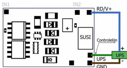
Aansluiting van een buffercircuit volgens RCN-530 (bijv. UPS-mini)
