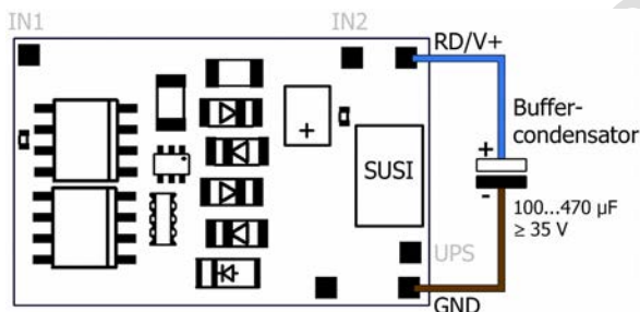
Aansluiting van een back-up condensator
