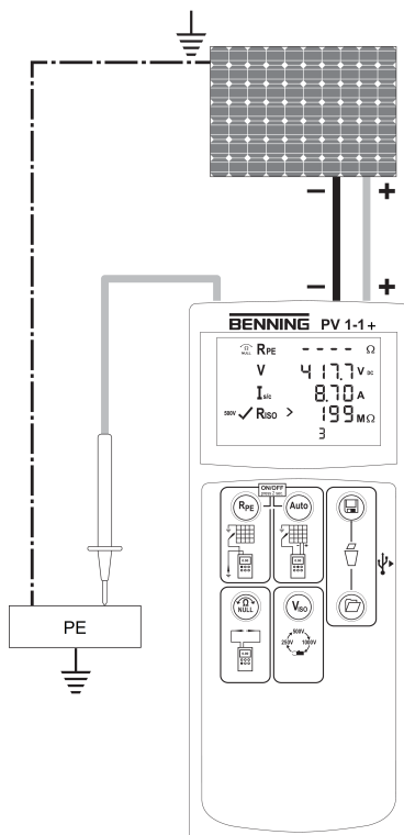
Afbeelding 5: Automatische fotovoltatische meting
