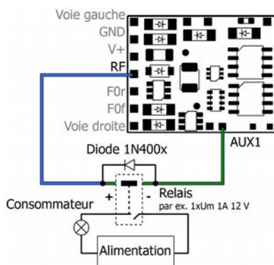
Connexion d'un consommateur via un relais
