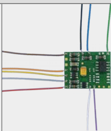
LD-W-42.2 avec câbles de raccordement N° d'article 41-05481
