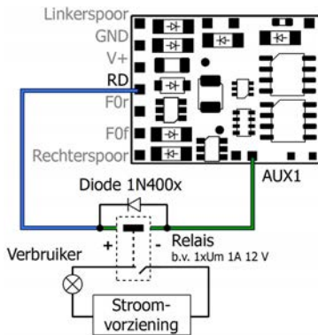
Aansluiten van een verbruiker via een relais
