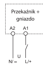
Schemat łączeniowy
