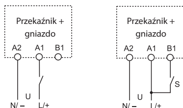
Schemat połączeń (bez sygnału START)
