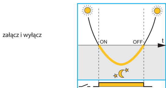
WYŁĄCZNIK ZMIERNY OSZCZĘDZAJĄCY ENERGIĘ TYP 11.41 (BEZ HISTEREZY)
