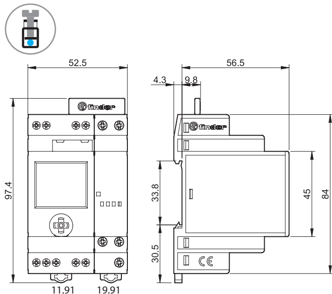
11.91 + 19.91 przełącznik mocy Zaciski śrubowe
