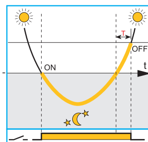
WYŁĄCZNIK ZMIERNY STANDARDOWY
