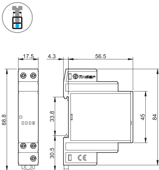
19.91 (przełącznik mocy do 11.91) Zaciski śrubowe
