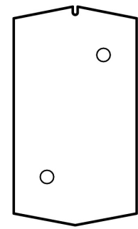
Ściana tylna: 2 x membrany przelotowe o Ø maks. 11 mm (nie dotyczy CI-K2H)
