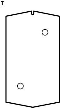
Ściana tylna: 2 x membrany przelotowe o Ø maks. 11 mm (nie dotyczy CI-K2H)
