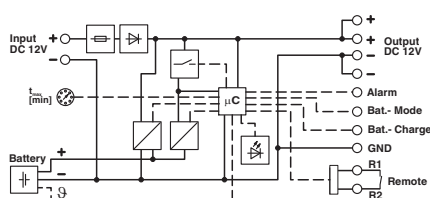
Schemat blokowy
