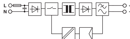
Schemat blokowy
