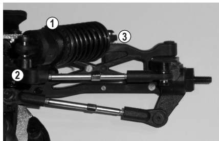
Oś przednia
