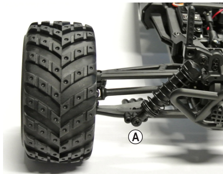
Rysunek 7: Oś przednia
