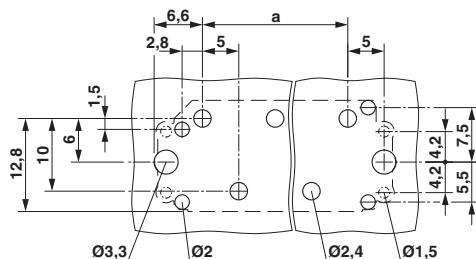
Szablon wierceń
