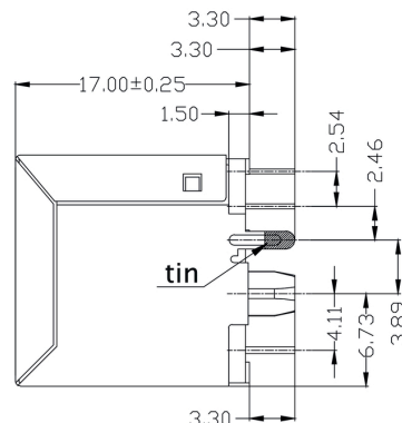
Rysunek wymiarowy
