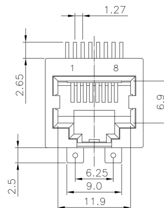
Rysunek wymiarowy
