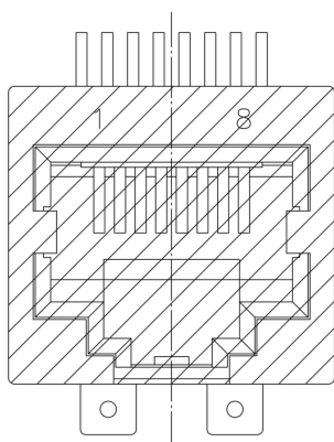
Rysunek wymiarowy
