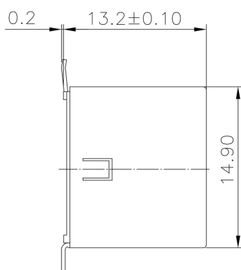
Rysunek wymiarowy
