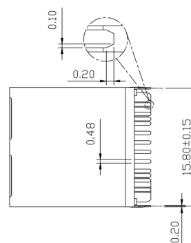
Rysunek wymiarowy
