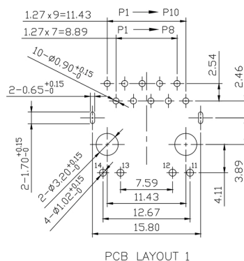
Układ płytek obwodu drukowanego
