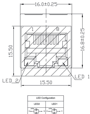
Rysunek wymiarowy
