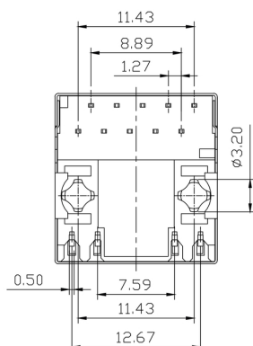
Rysunek wymiarowy
