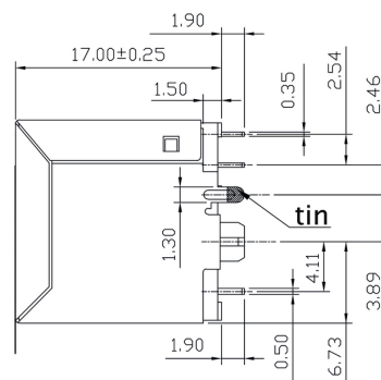
Rysunek wymiarowy
