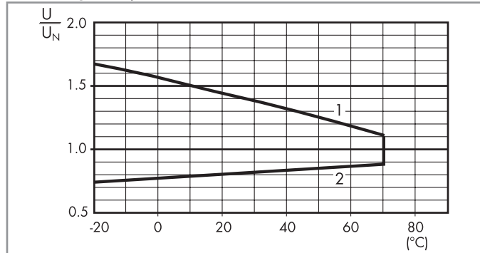
R 41 - AC Dopuszczalny zakres napięcia pracy cewki w zależności od temperatury otoczenia
