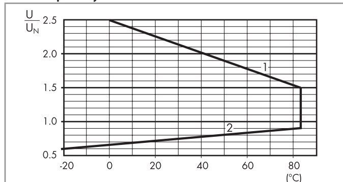
R 41 - DC Dopuszczalny zakres napięcia pracy cewki w zależności od temperatury otoczenia
