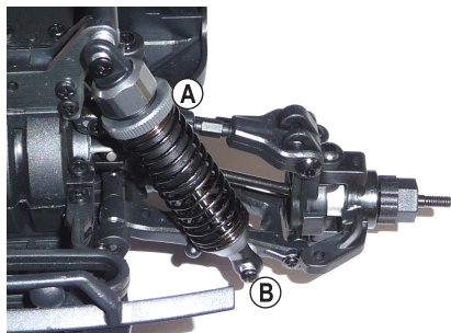
Oś przednia
