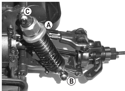
Oś tylna
