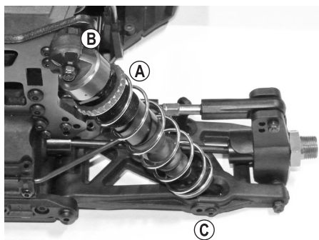
Assale posteriore
