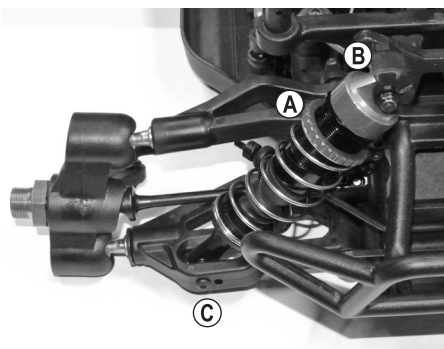
Assale anteriore
