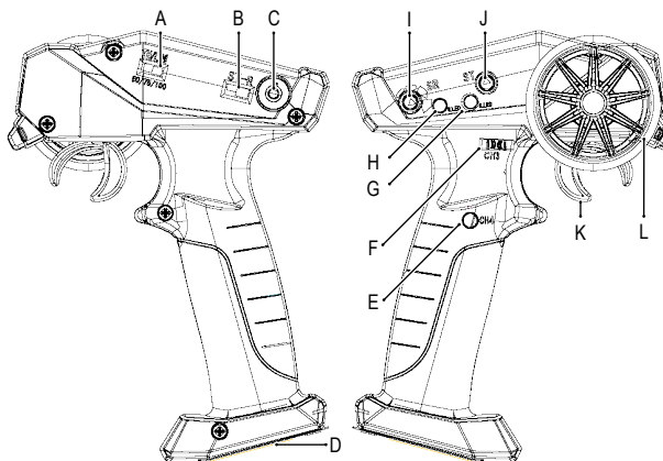
A 50/75/100: Snelheidsregeling
