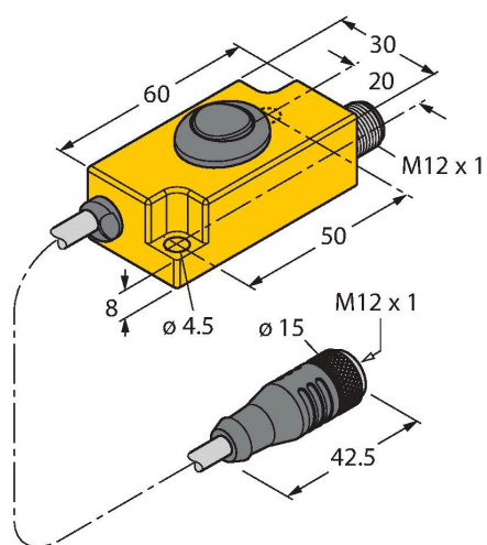
TX1-Q20L60
