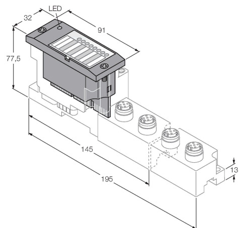
BL67-4IOL
