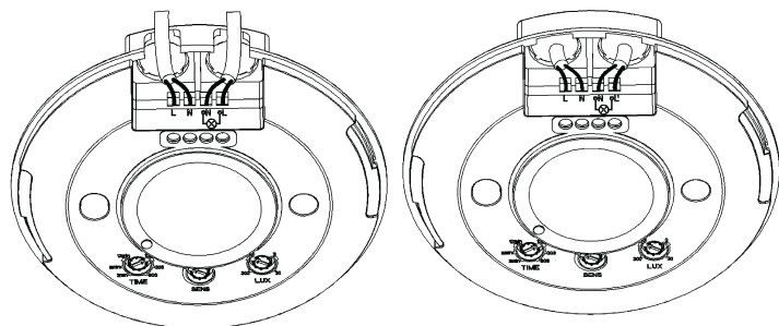
Schemat połączeń
