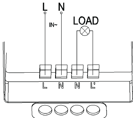
Schemat połączeń
