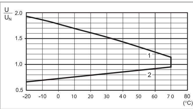
R 60 - Campo de operação da bobina DC versus temperatura ambiente
