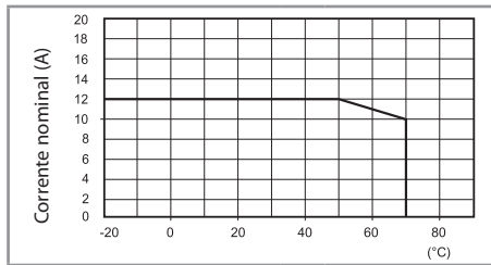
L 96 - Corrente nominal versus temperatura ambiente
