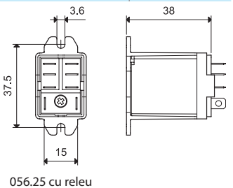
Adaptor de montare tip flanșă pe spatele releului pentru tipurile 55.32, 55.33, 55.34
