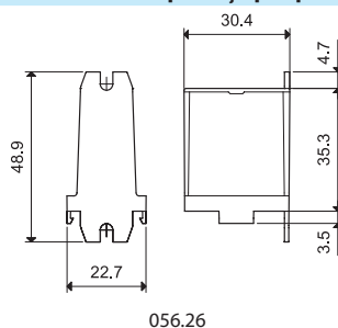
Adaptor de montare pe șină de 35 mm (EN 60715) pentru tipurile 55.32, 55.33, 55.34
