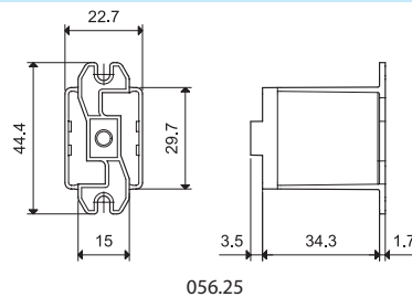
Adaptor de montare tip flanșă pe spatele releului pentru tipurile 55.32, 55.33, 55.34
