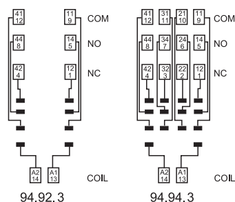
Terminalele de jos
