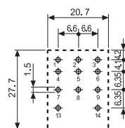
Vedere de jos (pe partea pinilor)
