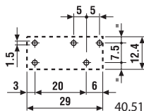
Вид со стороны выводов
