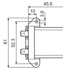
Фланцевый адаптер крепления для типов 62.3х и 62.8х.хххх.ххх9
