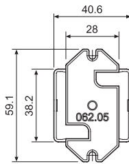
Фланцевый адаптер крепления для типов 62.3х и 62.8х.хххх.ххх9
