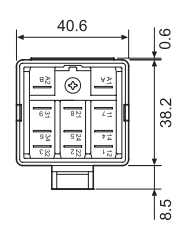
Адаптер для 35 мм рейки (EN 60715) для типов 62.3х и 62.8х.хххх.ххх9
