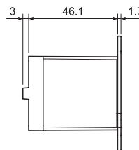
Адаптер для 35 мм рейки (EN 60715) для типов 62.3х и 62.8х.хххх.ххх9
