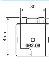
Адаптер для 35 мм рейки (EN 60715) для типов 62.3х и 62.8х.хххх.ххх9
