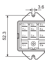
Адаптер для 35 мм рейки (EN 60715) для типов 62.3х и 62.8х.хххх.ххх9
