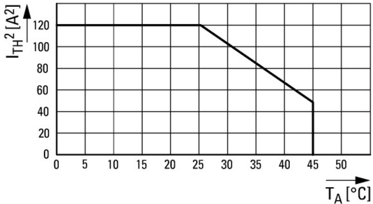
Кривая дерейтинга
