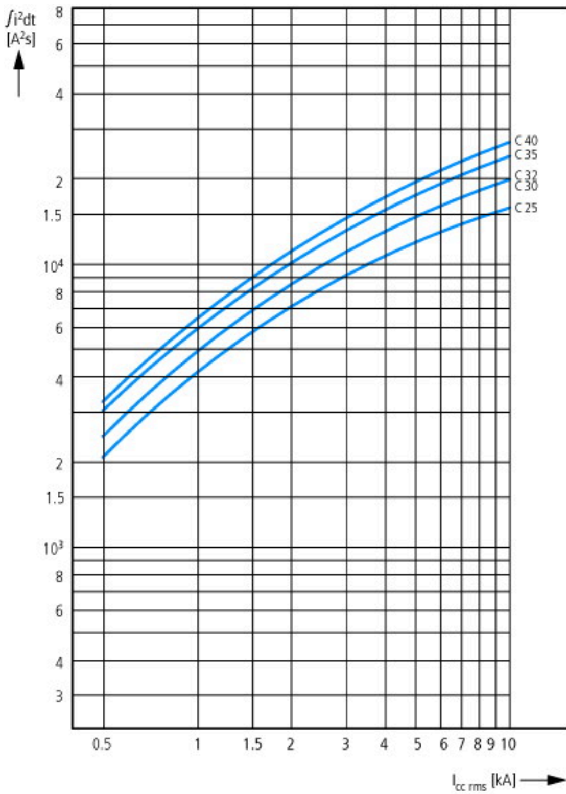
Характеристика С (25 - 40 А), 240 В
