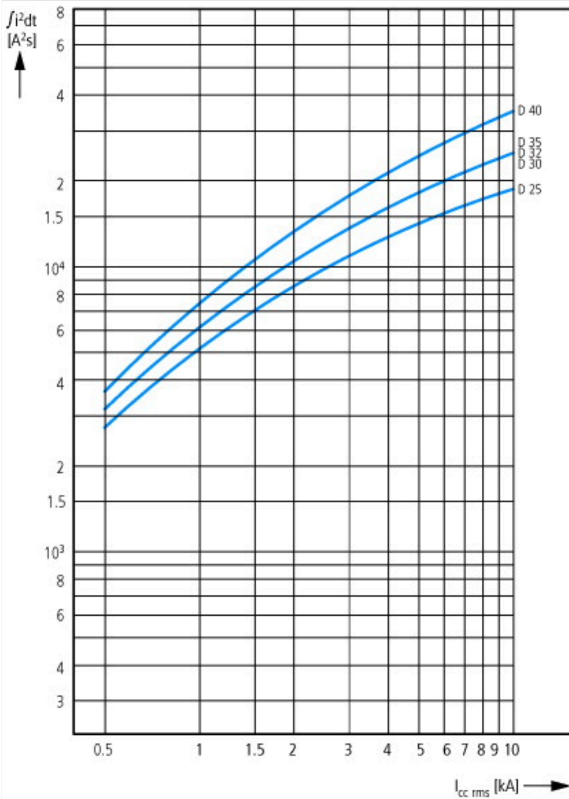
Характеристика D (25 - 40 A), 240 В
