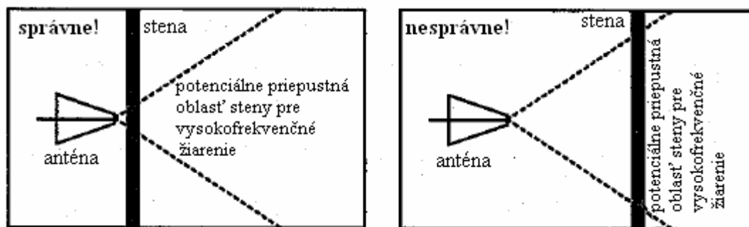
obrázok: ilustračný náčrt umiestnenia meracej antény
