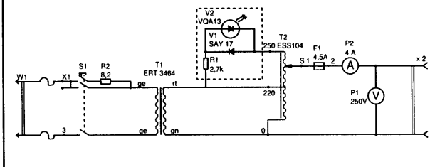
Regulační auto transformátor LTS 604
