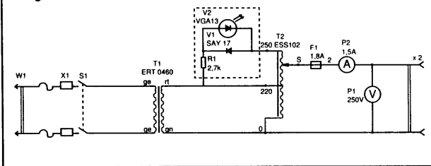
Regulační auto transformátor LTS 602
