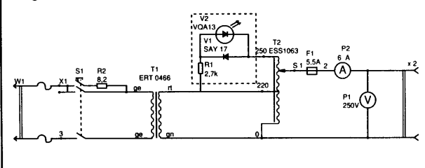
Regulační auto transformátor LTS 606
