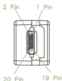
Moška vtičnica za monitor (vhod)
