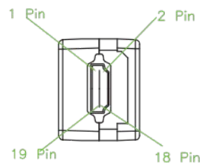
Ženski HDMI (izhod)
