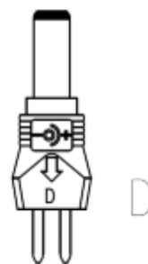
Koaksialni vtič Ø 2,1 x Ø 5 x 12 mm
