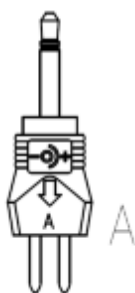
Banana vtič Ø 2,5 x 13 ±0,5 mm
