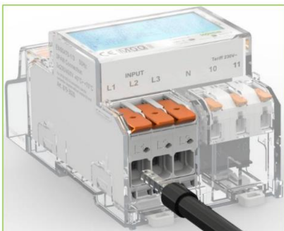
Shema ožičenja: Finožični vodnik z izoliranim zaključnim tulcem
