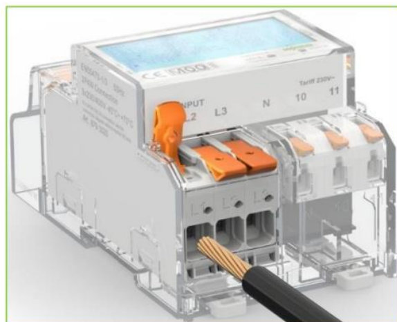
Shema ožičenja: Finožični vodnik
