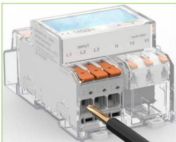
Shema ožičenja: Trdi vodnik
