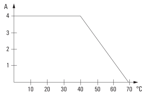
DC-lastgränskurva
