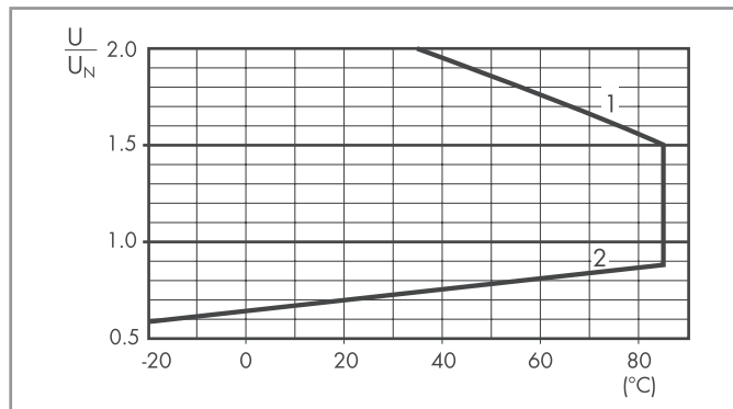
R 34 - DC 線圈操作範圍與環境溫度
