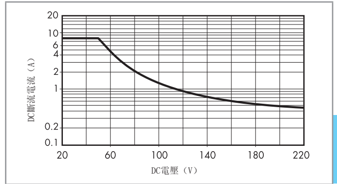
H 50 - 最大DC1斷流量 (類型 50.14)
