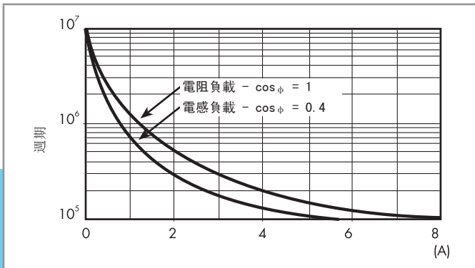
F 50 - 電氣壽命 (AC) 對比觸點電流 (類型 50.12)
