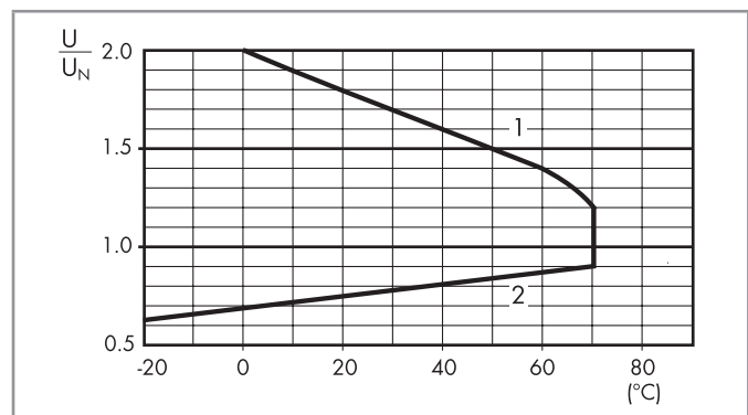
R 50 - DC線圈工作範圍對比環境溫度 標準線圈 (類型 50.12)
