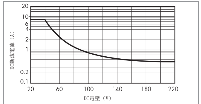
H 50 - 最大DC1斷流量 (類型 50.16)
