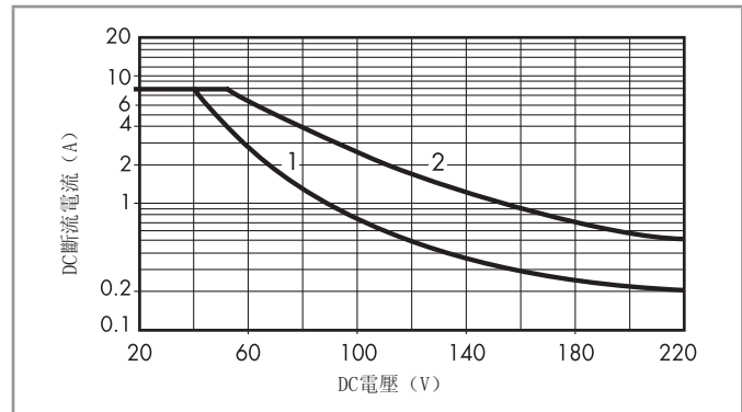
H 50 - 最大DC1斷流容量 (類型 50.12)
