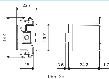
後方法蘭安裝轉接器，適用於55.32、55.33、55.34
