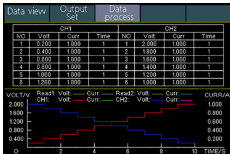
Programmierte Spannungsausgabe auf Kanal 1 und Kanal 2.
