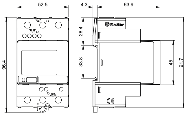
Typ 7M.38.8.400.0112
