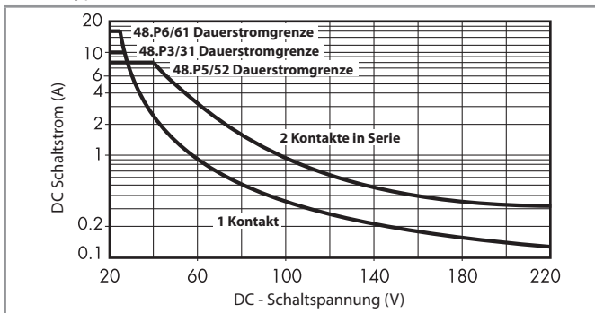
H 48 - Gleichstromschaltvermögen bei DC1 - Belastung
