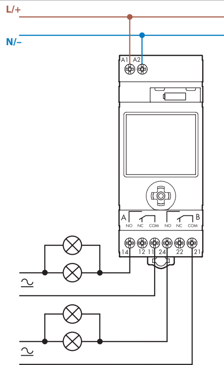
Typ 12.62 12.A2
