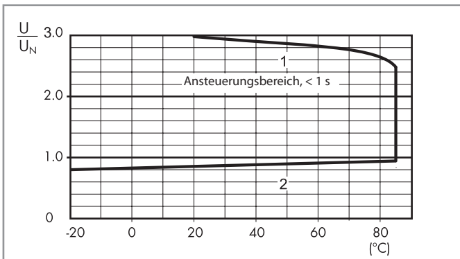
R 68-2 - Kurzzeitige DC Spulen-Ansteuerung, im Energiesparmodus mit Haltespannung bei (-40...+85)°C
