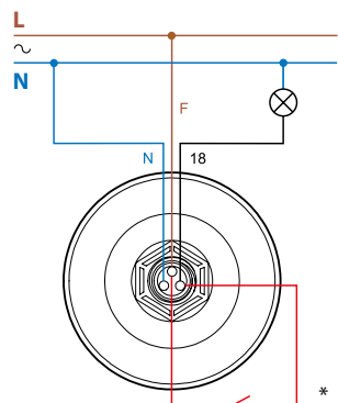
Typ 10.61
