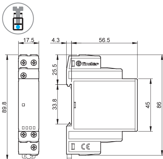
Typ 70.61 Schraubklemmen
