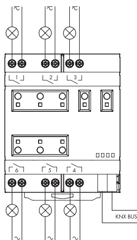
Typ 19.6K
