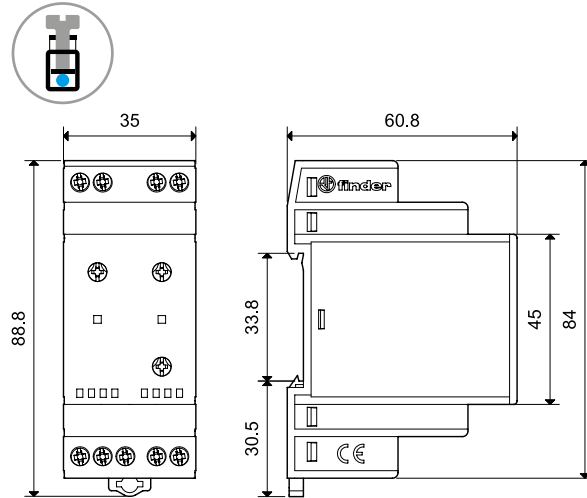
Typ 11.42 Schraubklemmen
