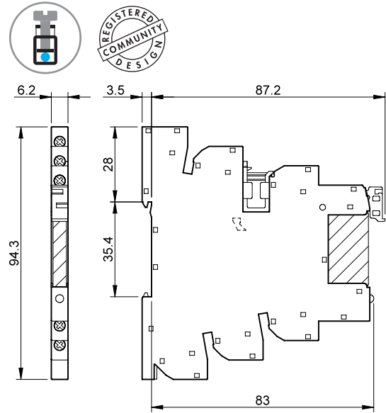
Typ 39.30/39.30.3 39.31/39.31.3 Schraubklemmen
