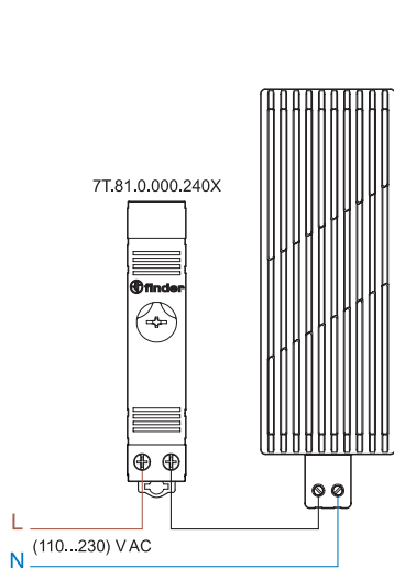
AC-Ausführung
