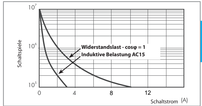
F 48 - Elektrische Lebensdauer bei AC
