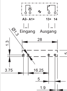
Ansicht auf die Anschlüsse
