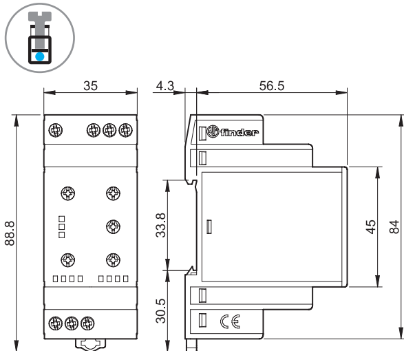
Typ 70.41 Schraubklemmen
