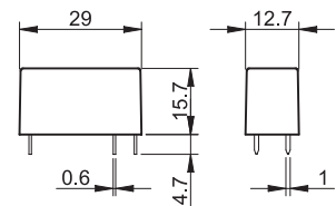
Typ 41.81-9024/41.81-8240
