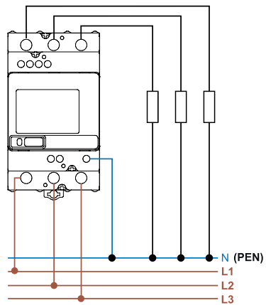
Typ 7M.38.8.400.0112
