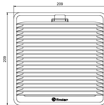
Typ 7F.02.0.000.3000
