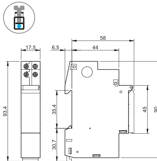
12.11 Schraubklemmen
