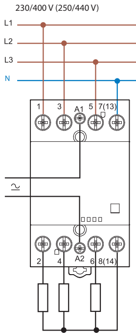
Typ 22.44/22.64
