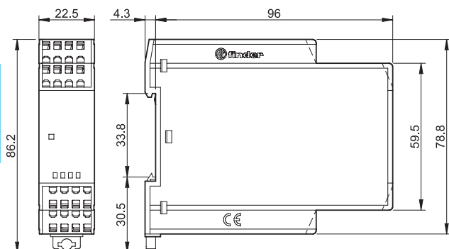
Typ 75.32 Schraubklemmen
