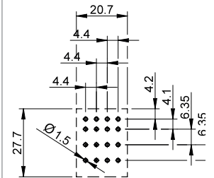
Ansicht auf die Anschlüsse
