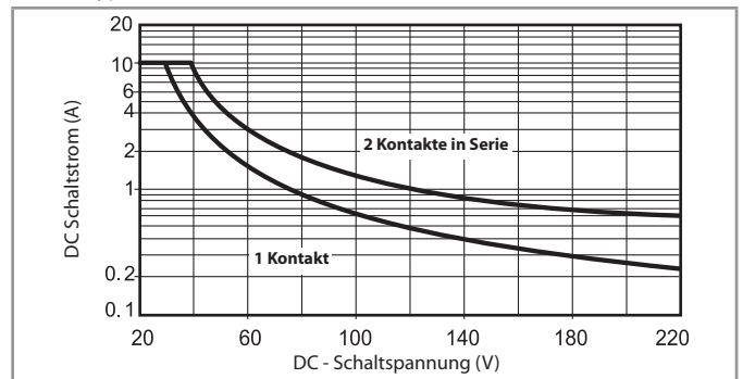
H 48 - Gleichstromschaltvermögen bei DC1 - Belastung
