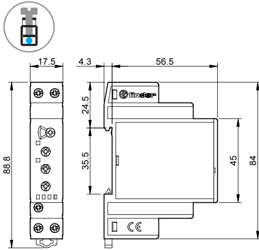
Typ 70.11 Schraubklemmen
