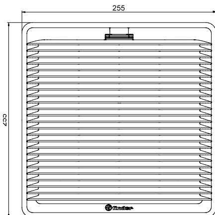
Typ 7F.20.x.xxx.4250
