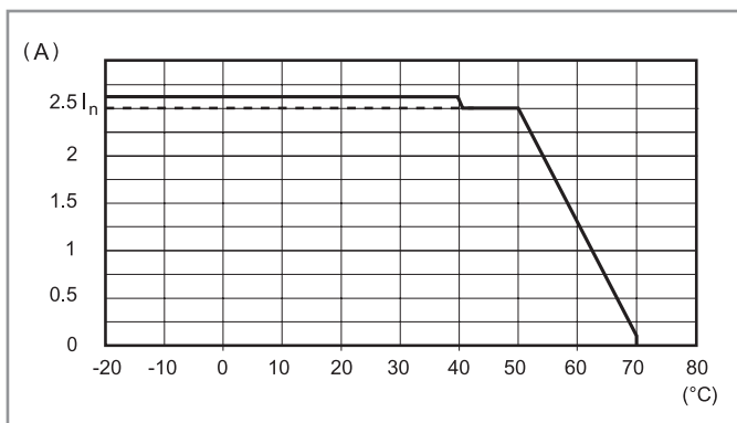
L78-6 Dauerstrom-Belastbarkeit (78.61)
