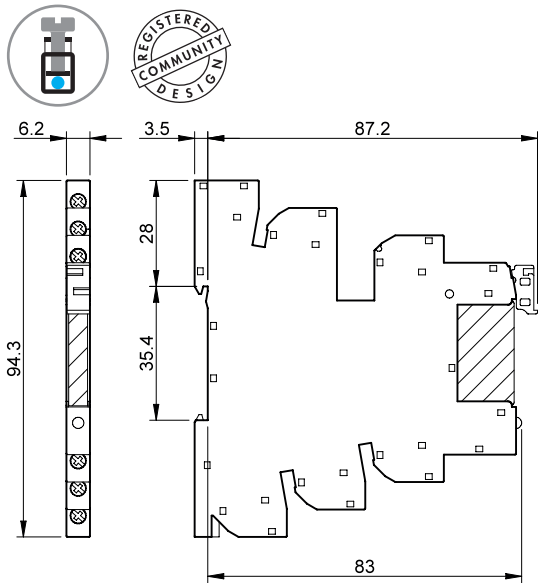
Typ 39.40 39.41 Schraubklemmen
