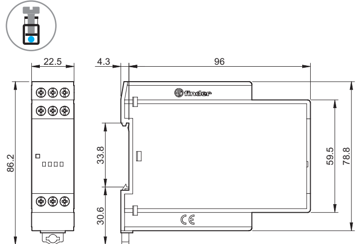
Typ 70.62 Schraubklemmen
