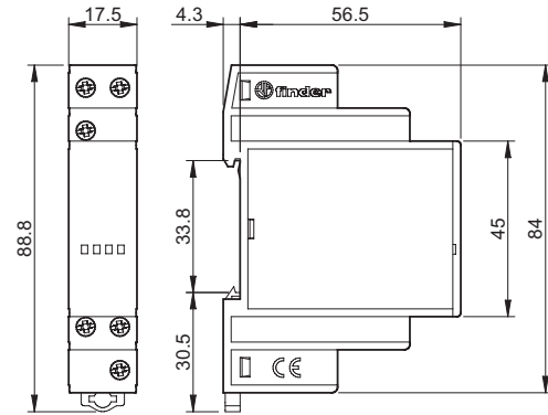
Typ 13.31/13.91 Schraubklemmen
