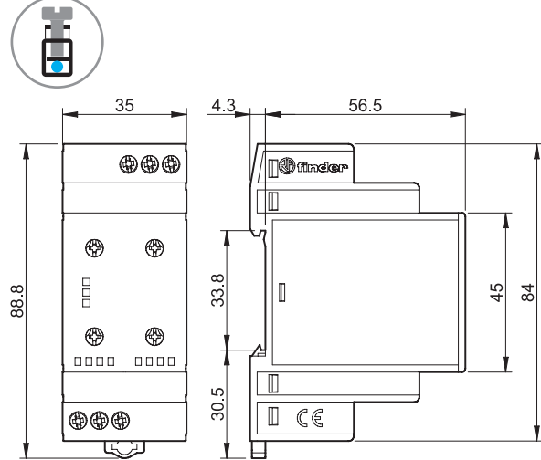
Typ 70.31 Schraubklemmen
