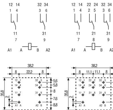
62.22 Ansicht auf die Anschlüsse 62.23 Ansicht auf die Anschlüsse
