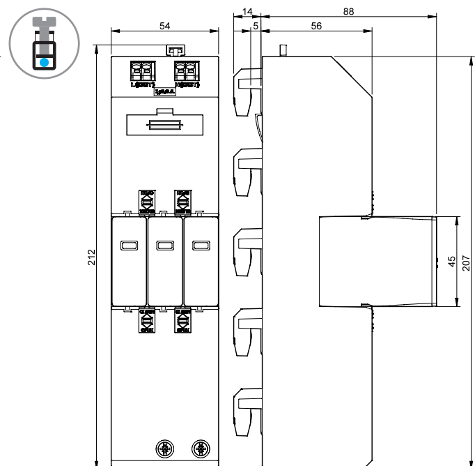
Typ 7P.04.8.255.Z0xx Schraubklemmen
