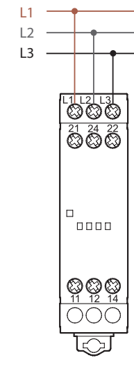
Typ 70.62
