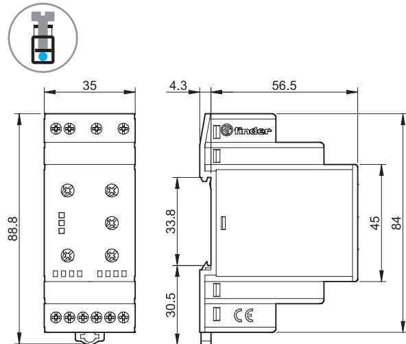
Typ 70.42 Schraubklemmen
