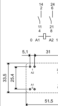
Ansicht auf die Anschlüsse
