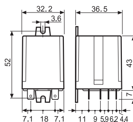
Typ 60.62
