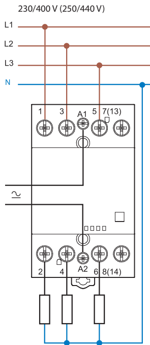
Typ 22.44/22.64
