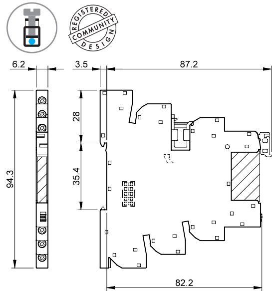
Typ 39.80 39.81 Schraubklemmen
