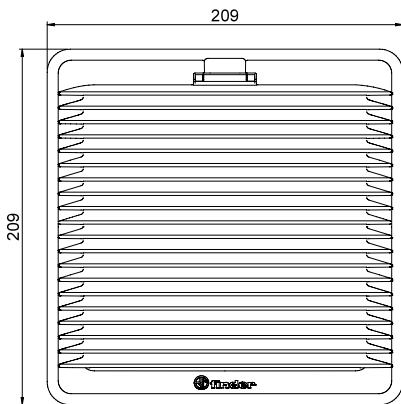
Typ 7F.20.x.xxx.3100
