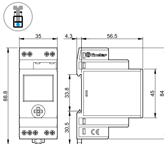
Typ 11.91 + 19.91 (Dämmungsschalter mit Brücke 011.19 + Ausgangsmodul) Schraubklemmen
