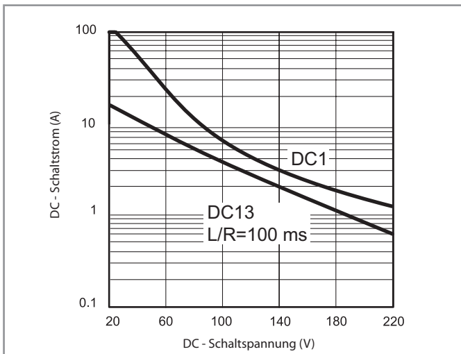
H 68 - Gleichstromschaltvermögen bei DC1- und DC13-Belastung
