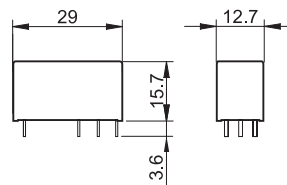
Typ 41.52.6.xxx/41.61.6.xxx
