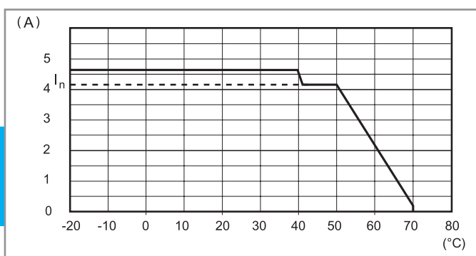
L78-5 Dauerstrom-Belastbarkeit (78.50/51)
