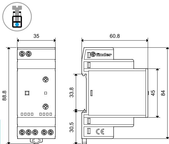
Typ 11.41 Schraubklemmen
