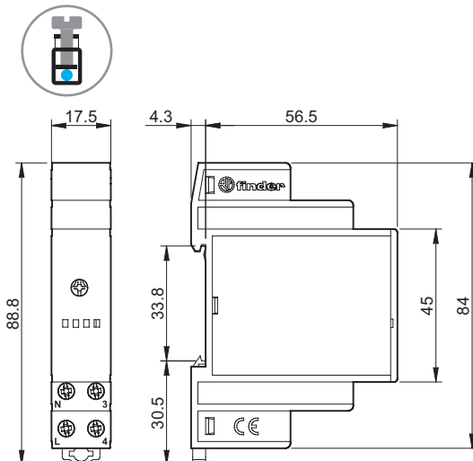
Typ 14.81 Schraubklemmen
