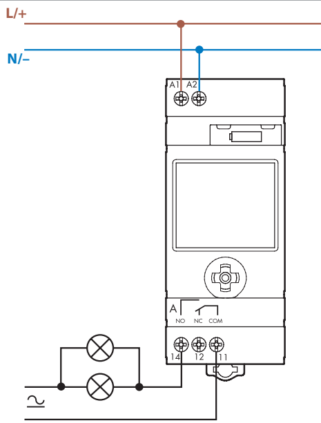
Typ 12.61 12.A1
