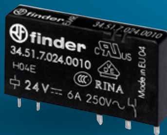
Schmales Steck-/Print-Relais, Serie 34 Best.-Nr. 502881-KI
