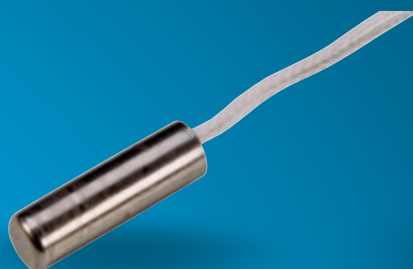
Platin-Temperatursensor im Edelstahlgehäuse Best.-Nr. 172412-KI
