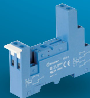
Zubehör für Serie 40, 41, 44: Serie 95 Best.-Nr. 502802-KI
